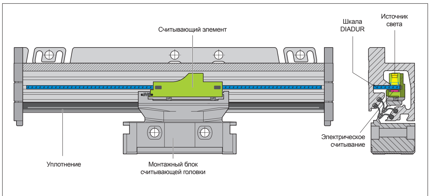
Схематическая конструкция закрытого датчика линейного перемещения LC 115
